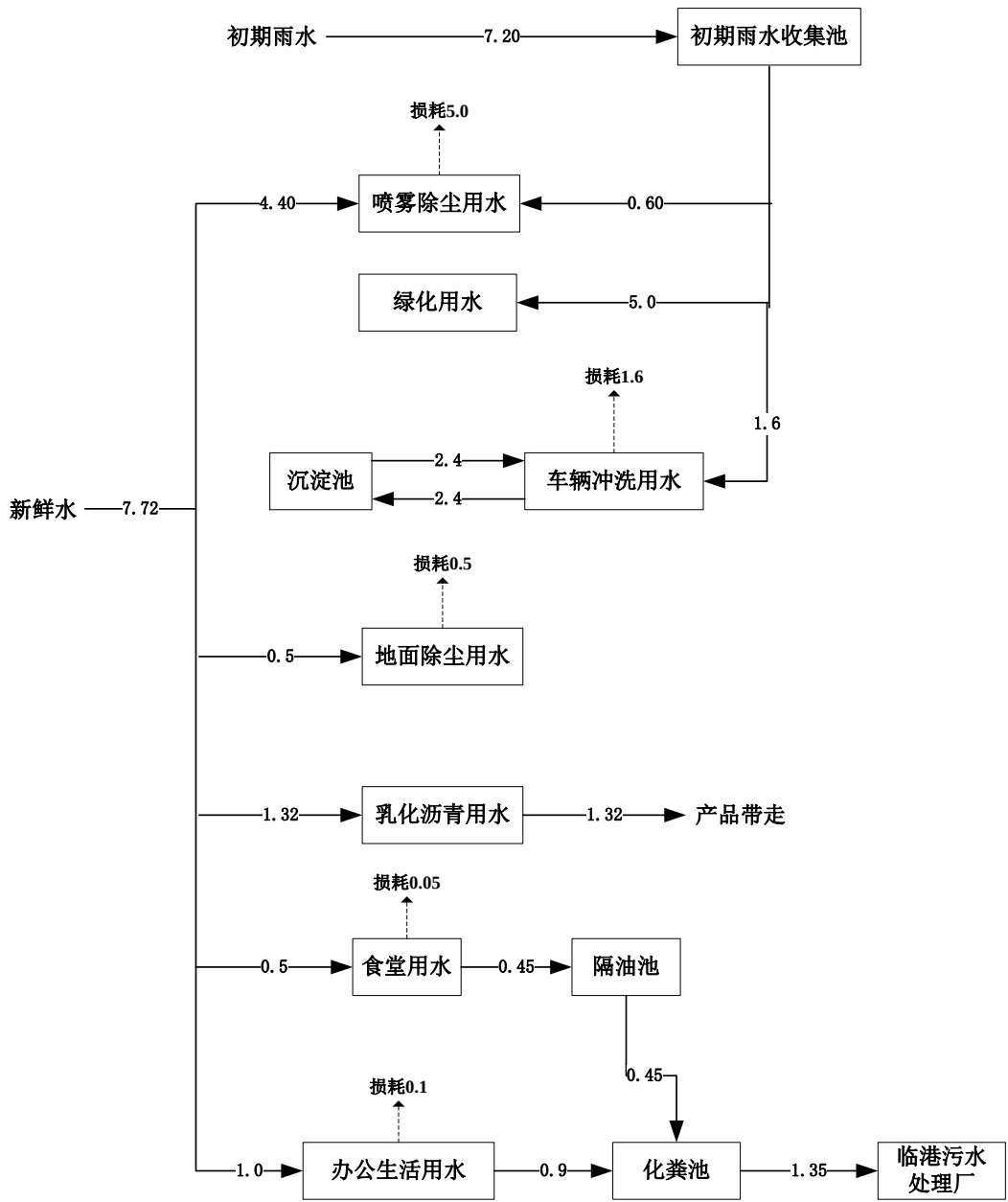
图2.1-1 本项目水平衡图 单位：m³/d
