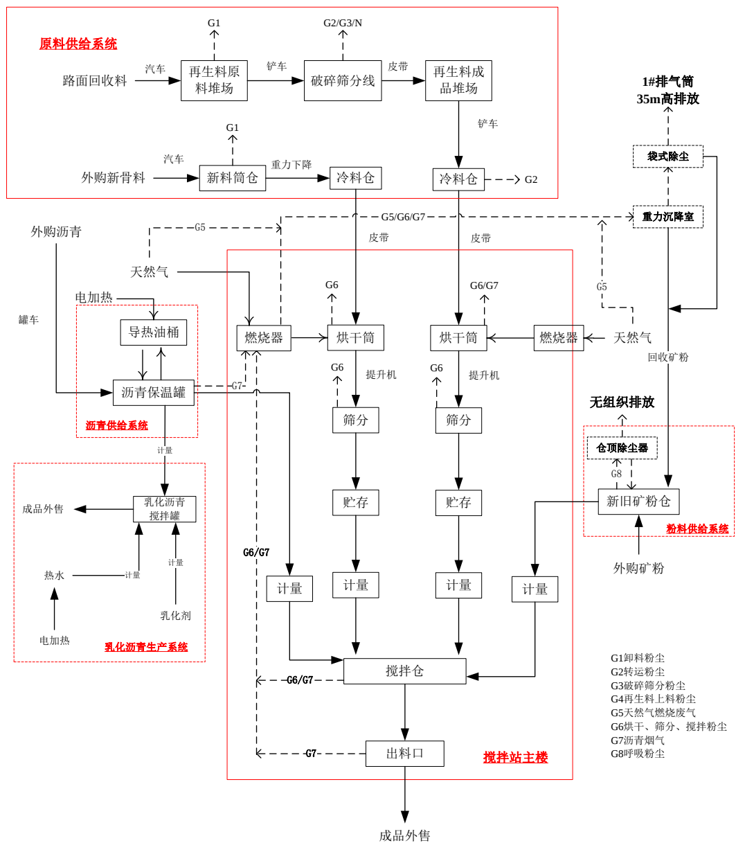
图2.2-1 沥青混凝土及乳化沥青生产工艺流程及产污环节图
