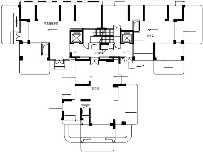
湖屿樾山二期6#楼 一层平面图
