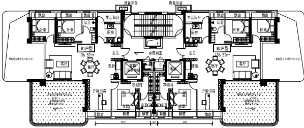
湖屿樾山二期6#楼 奇数层平面图
