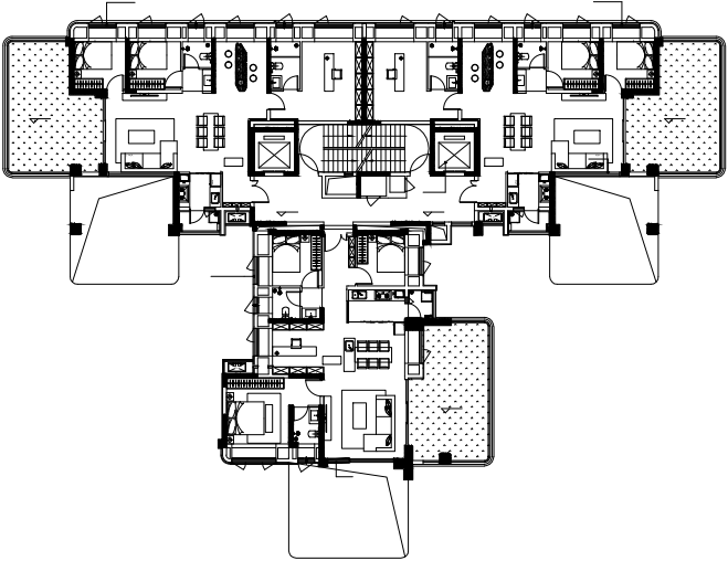
湖屿樾山二期6#楼 偶数层平面图
