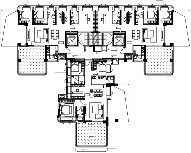
湖屿樾山二期6#楼 奇数层平面图
