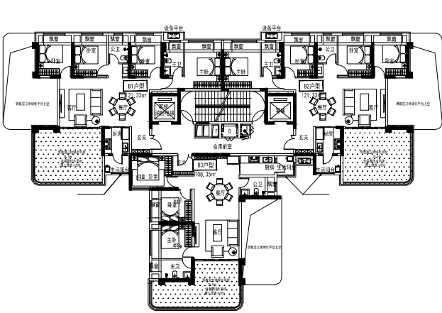
湖屿樾山二期4、5#楼 奇数层平面图
