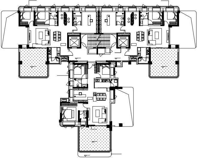
湖屿樾山二期4、5#楼 奇数层平面图
