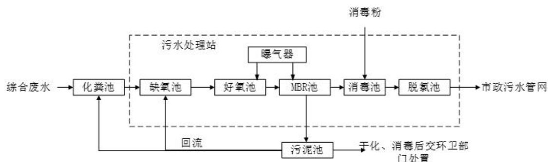
图 4-2 运营期污水处理站工艺流程图
