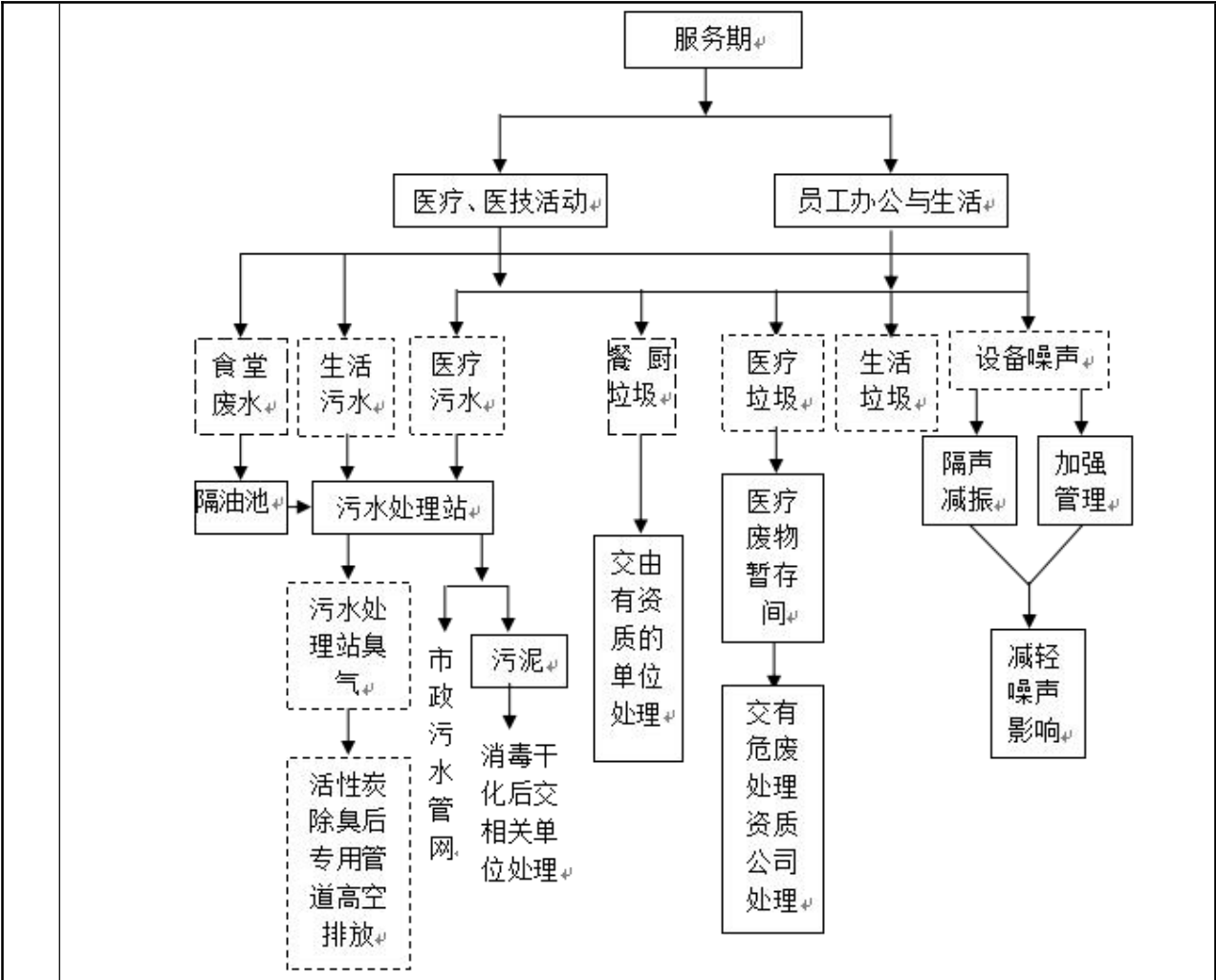
图 2-3 项目施工期工艺流程及产污环节图
