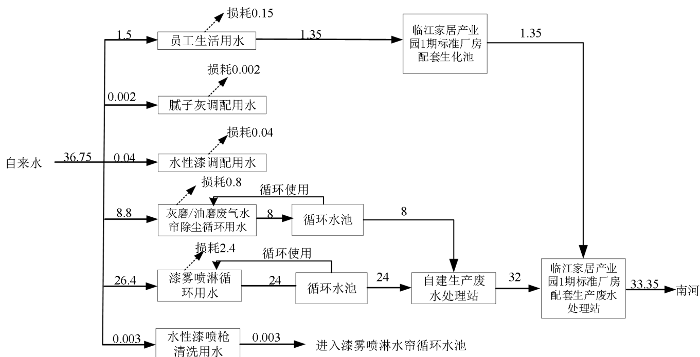
图 2.2-4 项目水平衡图（日最大用水）单位：m 3 /d
