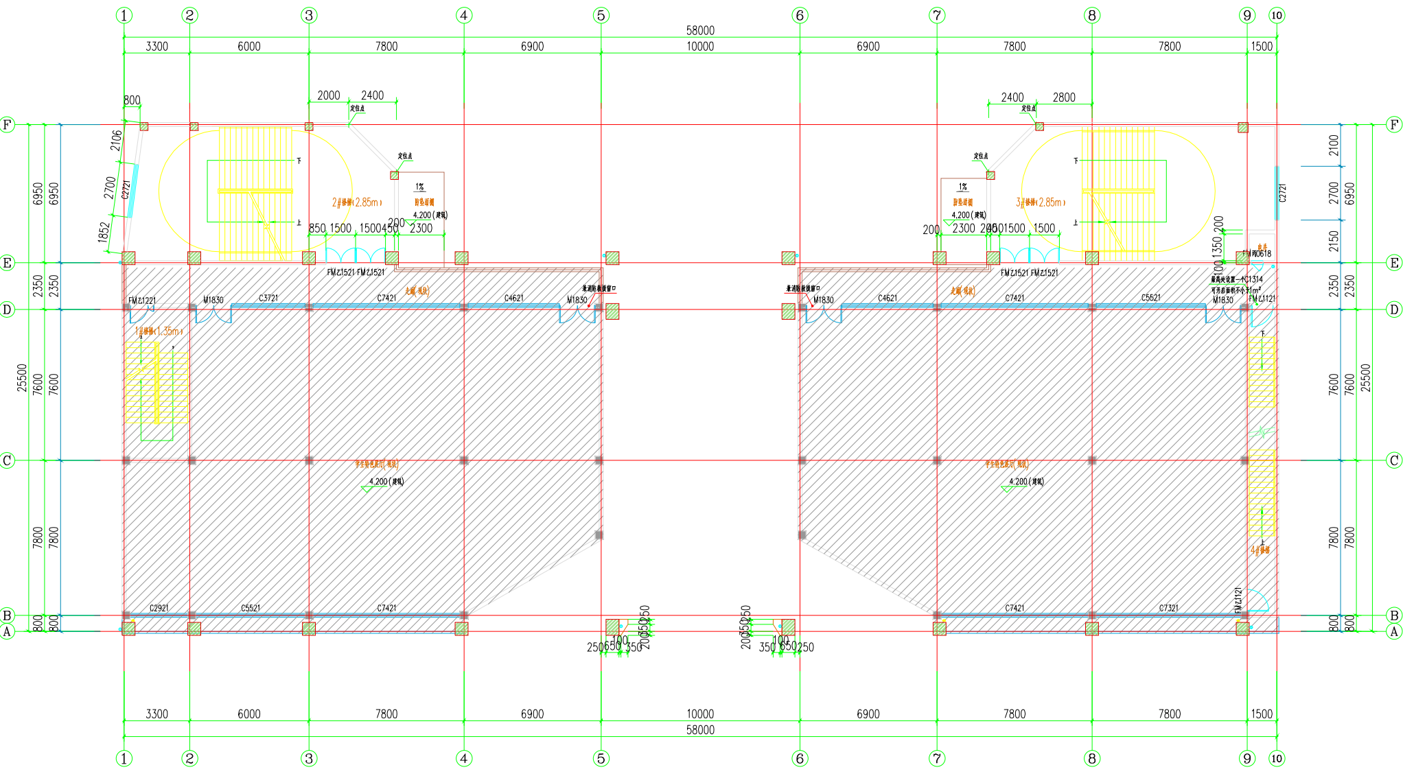
开州区龙珠中心小学功能室二层平面图
