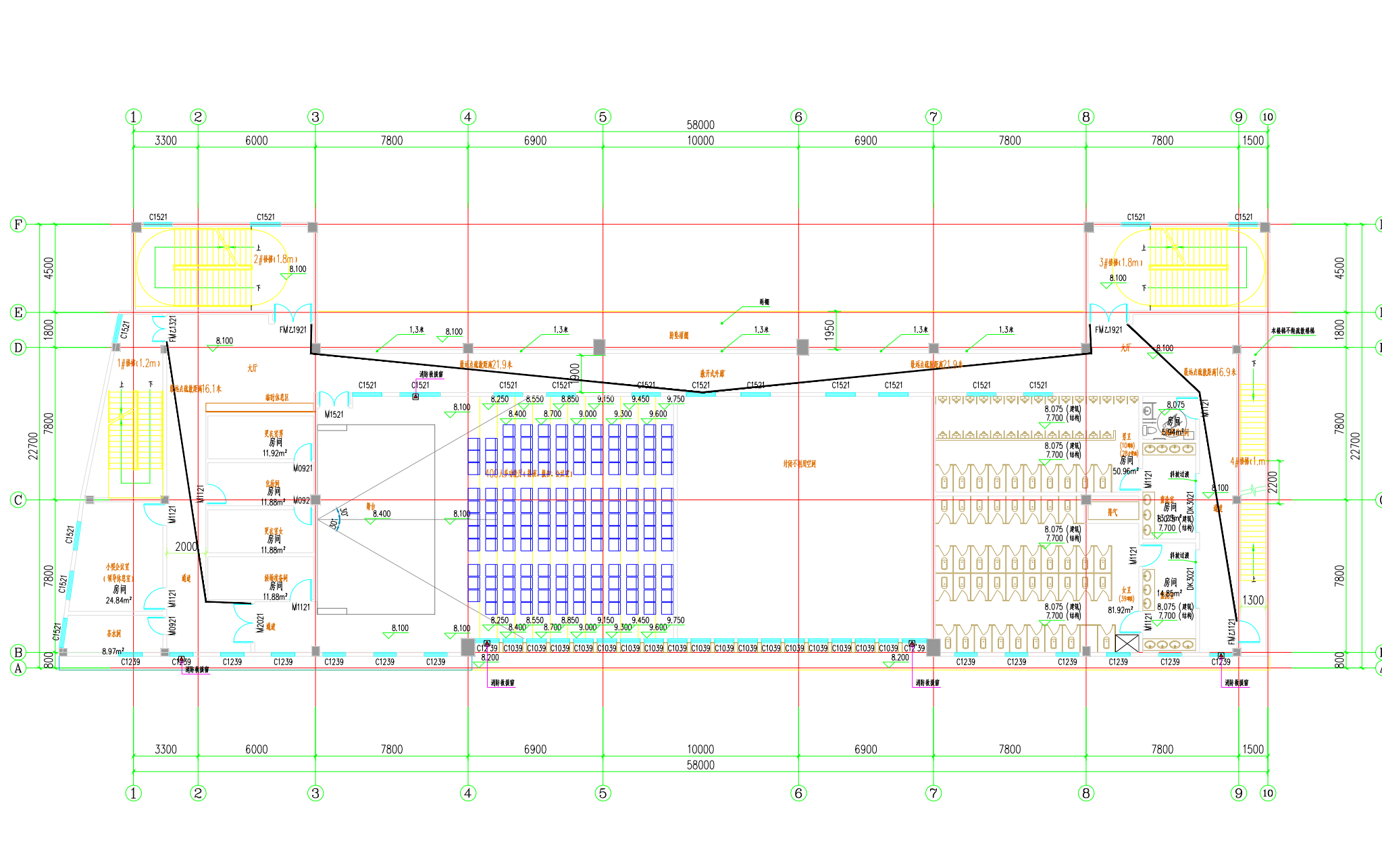
开州区龙珠中心小学功能室三层平面图
