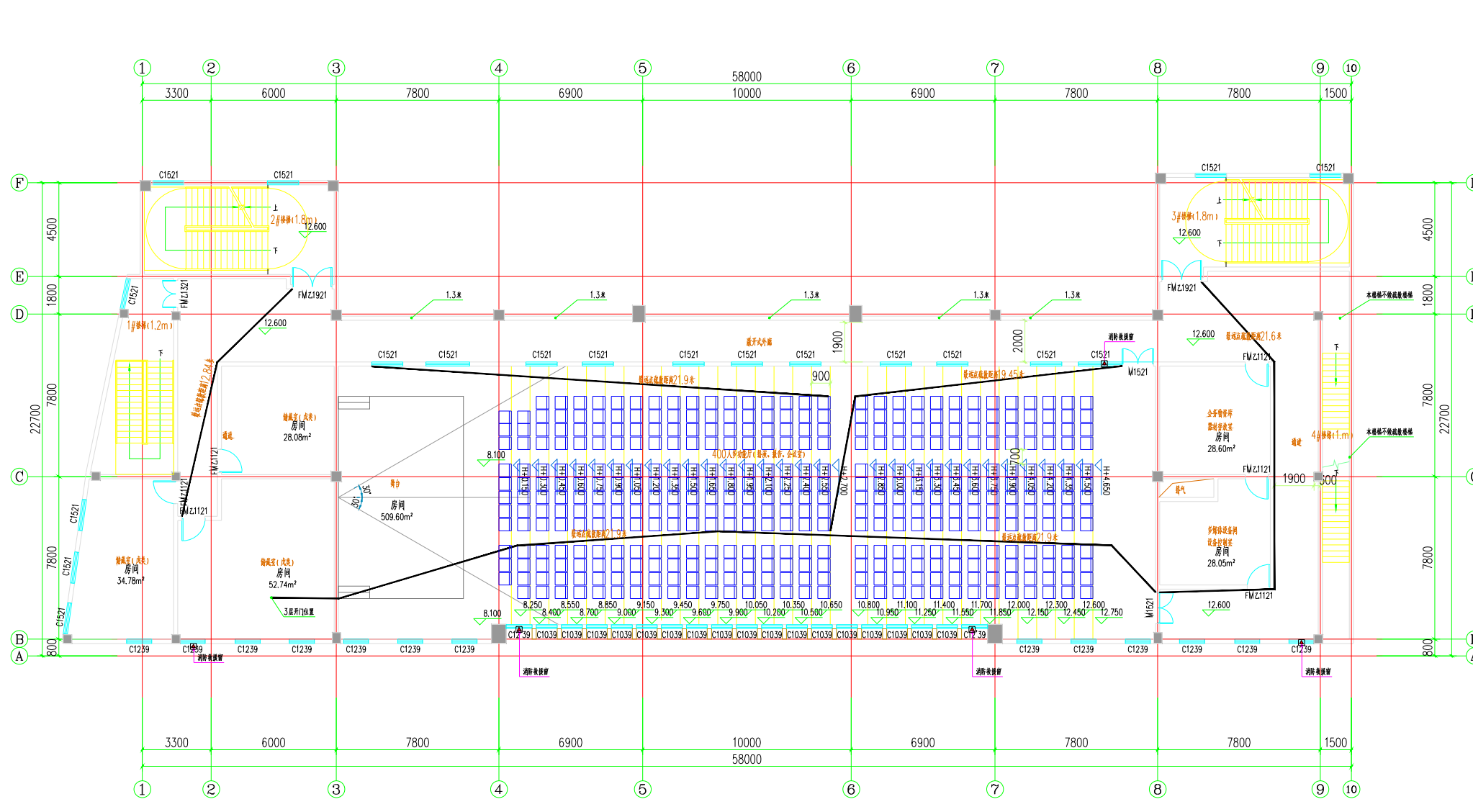
开州区龙珠中心小学功能室四层平面图
