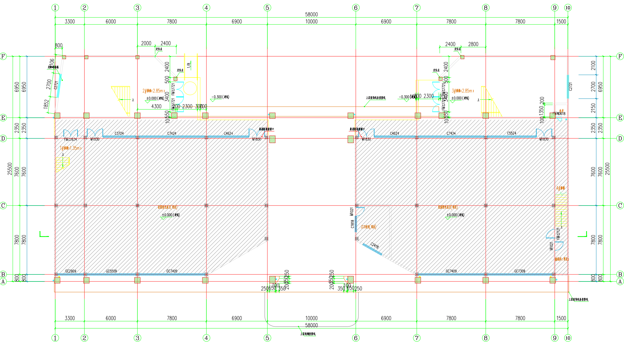
开州区龙珠中心小学功能室首层平面图
